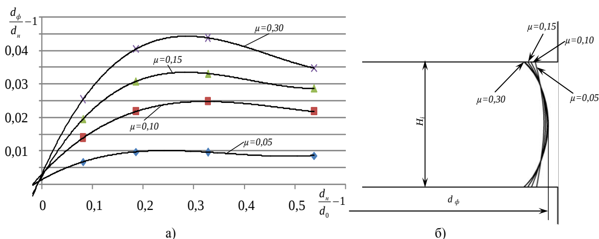
Рисунок 2.2 – Вплив номінального діаметру d_n зразка, що стискається, на його фактичний діаметру d_\phi при різних коефіцієнтах тертя \mu (а) і вплив коефіцієнта тертя на форму бічної поверхні стиснутого зразка (б)
