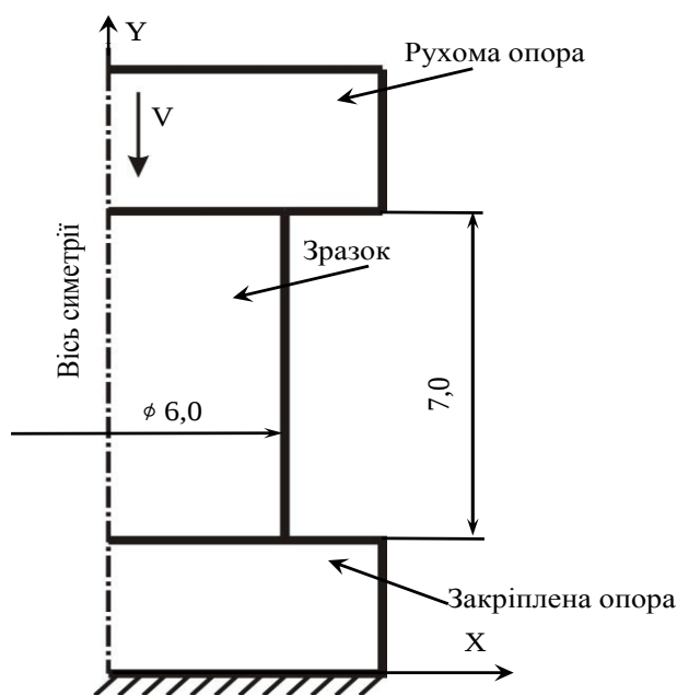
Рисунок 2.1 – Розрахункова схема дослідження на стискання
