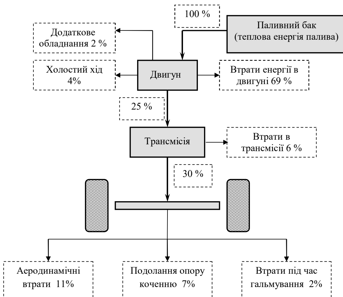
Рисунок 1.2 – Потіки відбору енергії пального під час експлуатації автомобіля у замиському циклі
