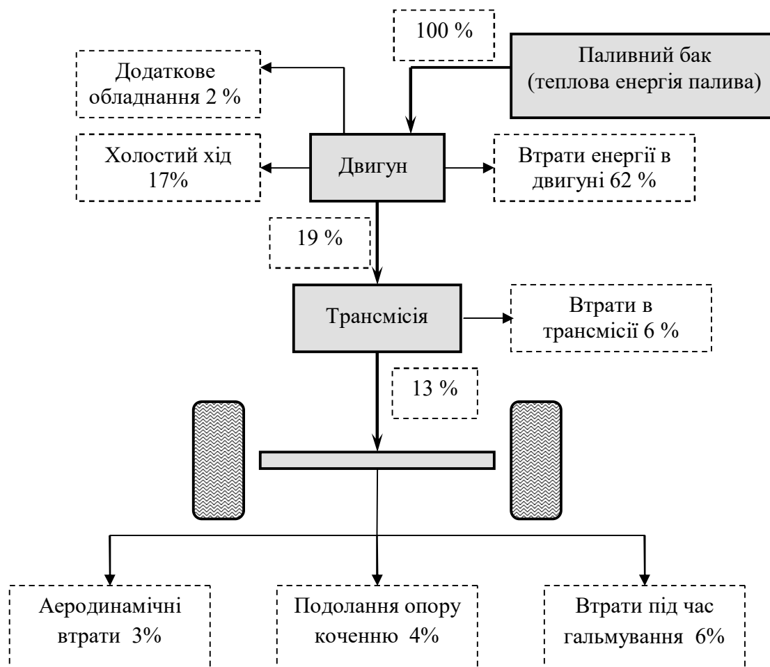
Рисунок 1.1 – Потіки відбору енергії пального під час експлуатації автомобіля у міському циклі
