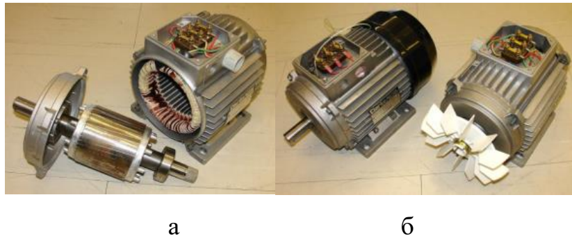
Рис. 5 – Система охолодження електродвигуна: а – природна; б – примусова
