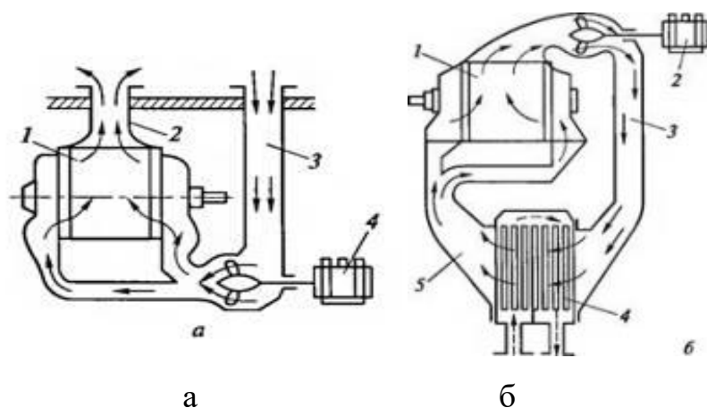
Рис. 7 – Незалежні системи вентиляції: а – розімкнена; б – замкнута
