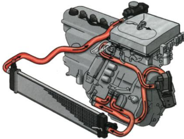
Рис. 8 – Система рідинного охолодження електроприводу Toyota
