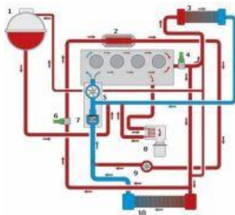
Рис. 2 – Система охолодження з системою рециркуляції відпрацьованих газів
