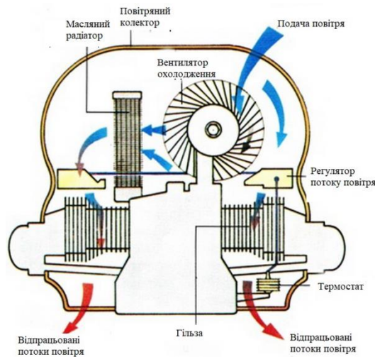
Рис. 4 – Система примусового повітряного охолодження
