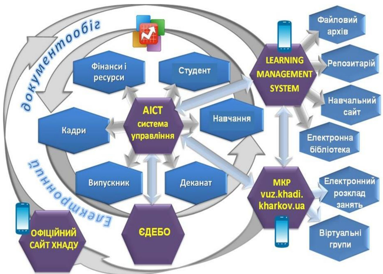
Рисунок 8.1 – Інформаційна система управління Університетом
