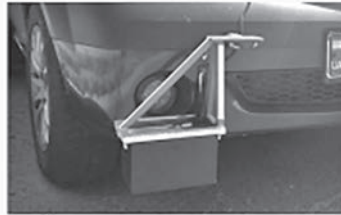
Установка лазерного сканування ЛВС 3.1-ХНАДУ (мобільний одноканальний лазерний профілограф)
